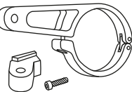
Käepideme kinnitus 35 mm Faceplate-adapter + kruvi
